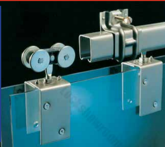
DOOR TRACK
